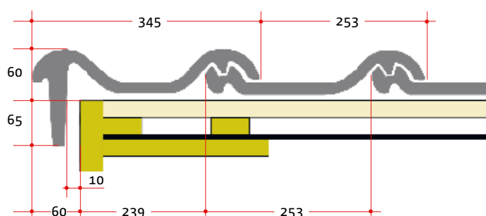
Ortgangausbildung mit Ortgangziegel links/rechts und Ortgangbrett Detail van gevelpan links/rechts met overstek en windveer Formation de l'avant-toit avec tuiles de rive droite/gauche et soffite d'avant-toit
